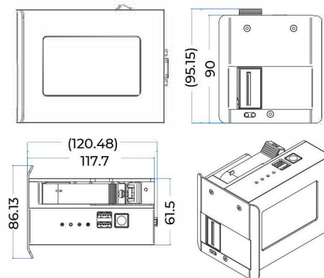
Smart-Jet® MAX
